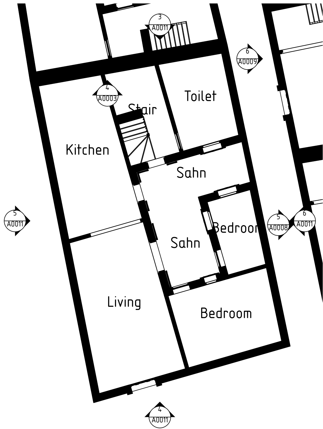
1 plot-9 0 1:100
