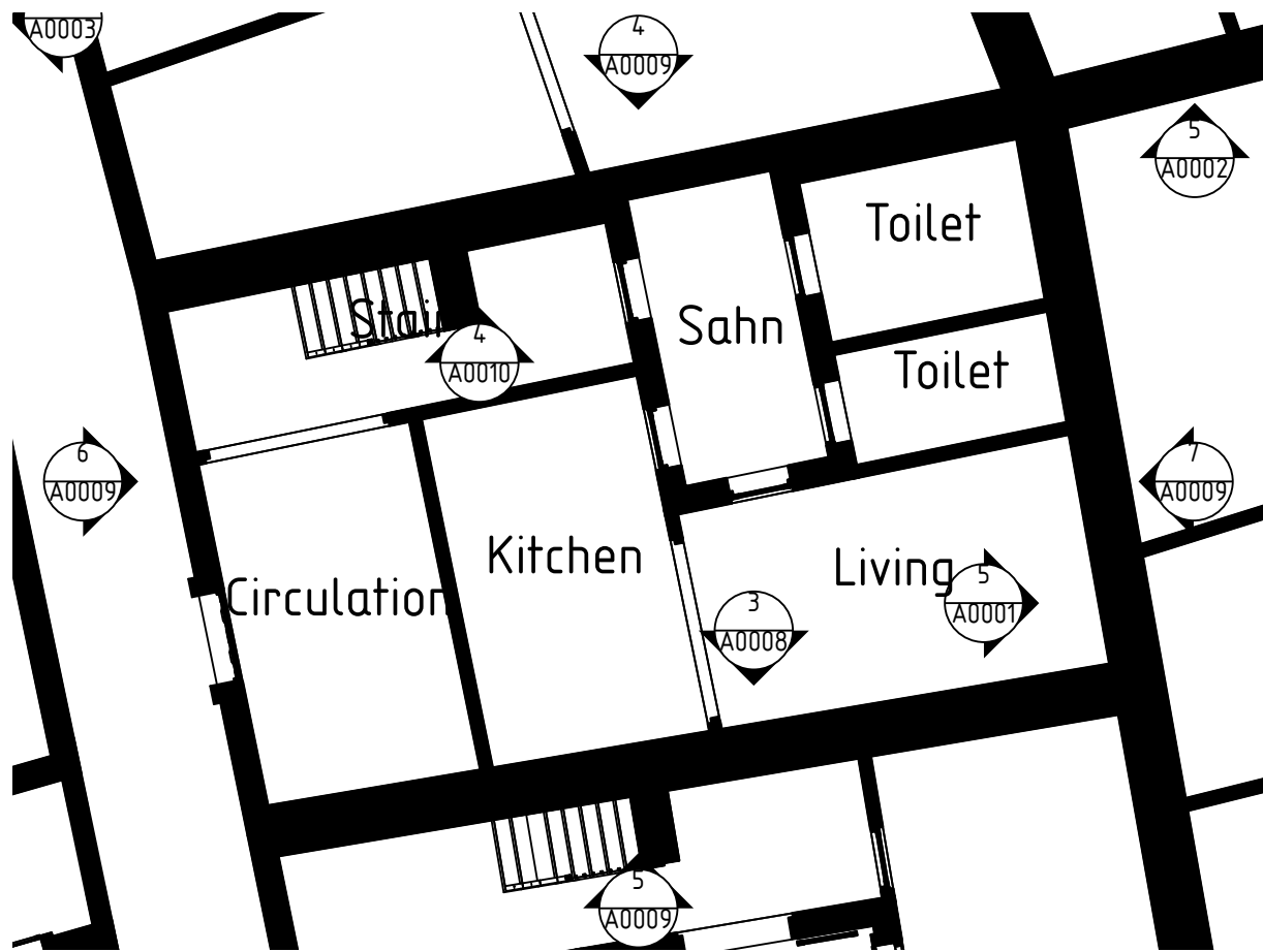
1 plot-7 0 1:100
