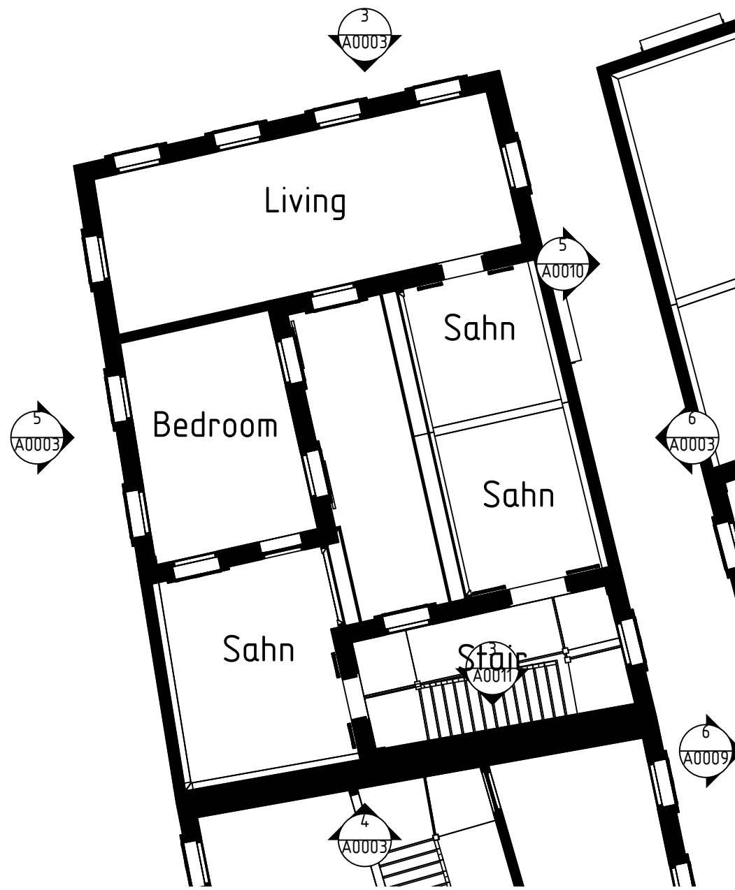
2 plot-10 1 1:100
