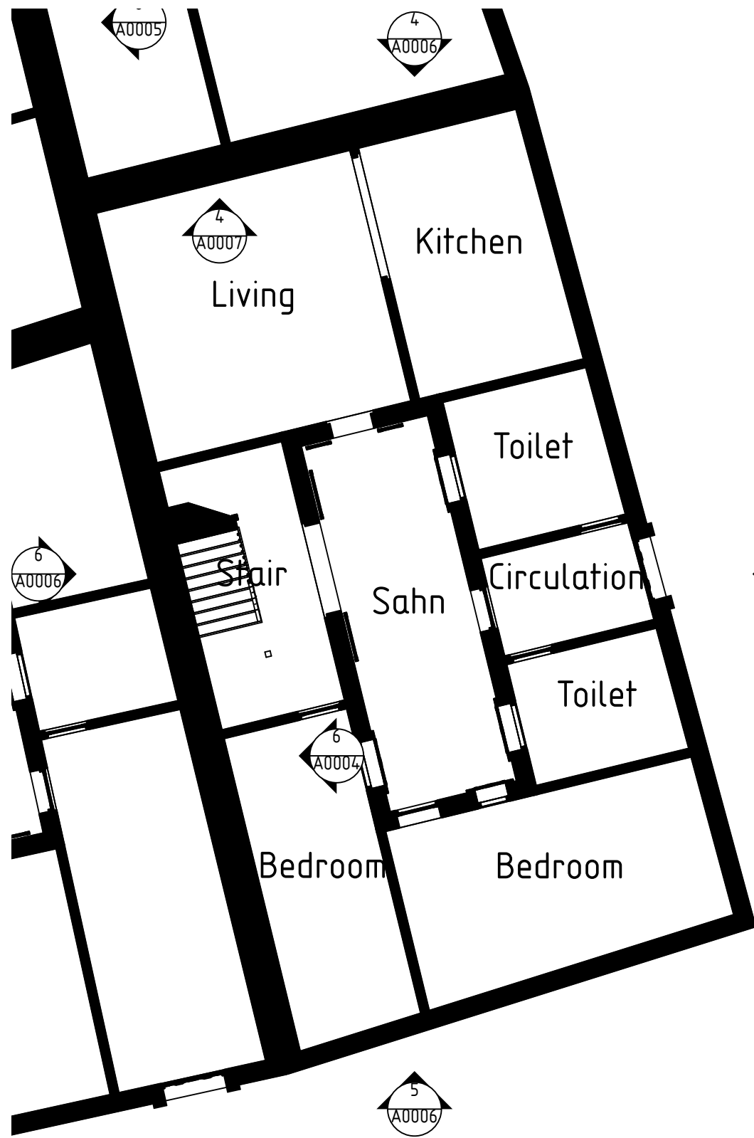
1 plot-4 0 1:100
