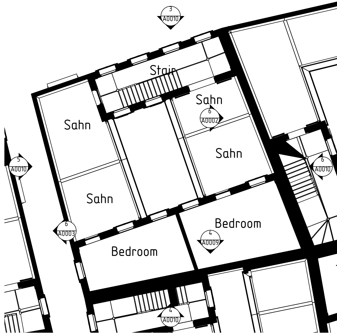
2 plot-8 1 1:100
