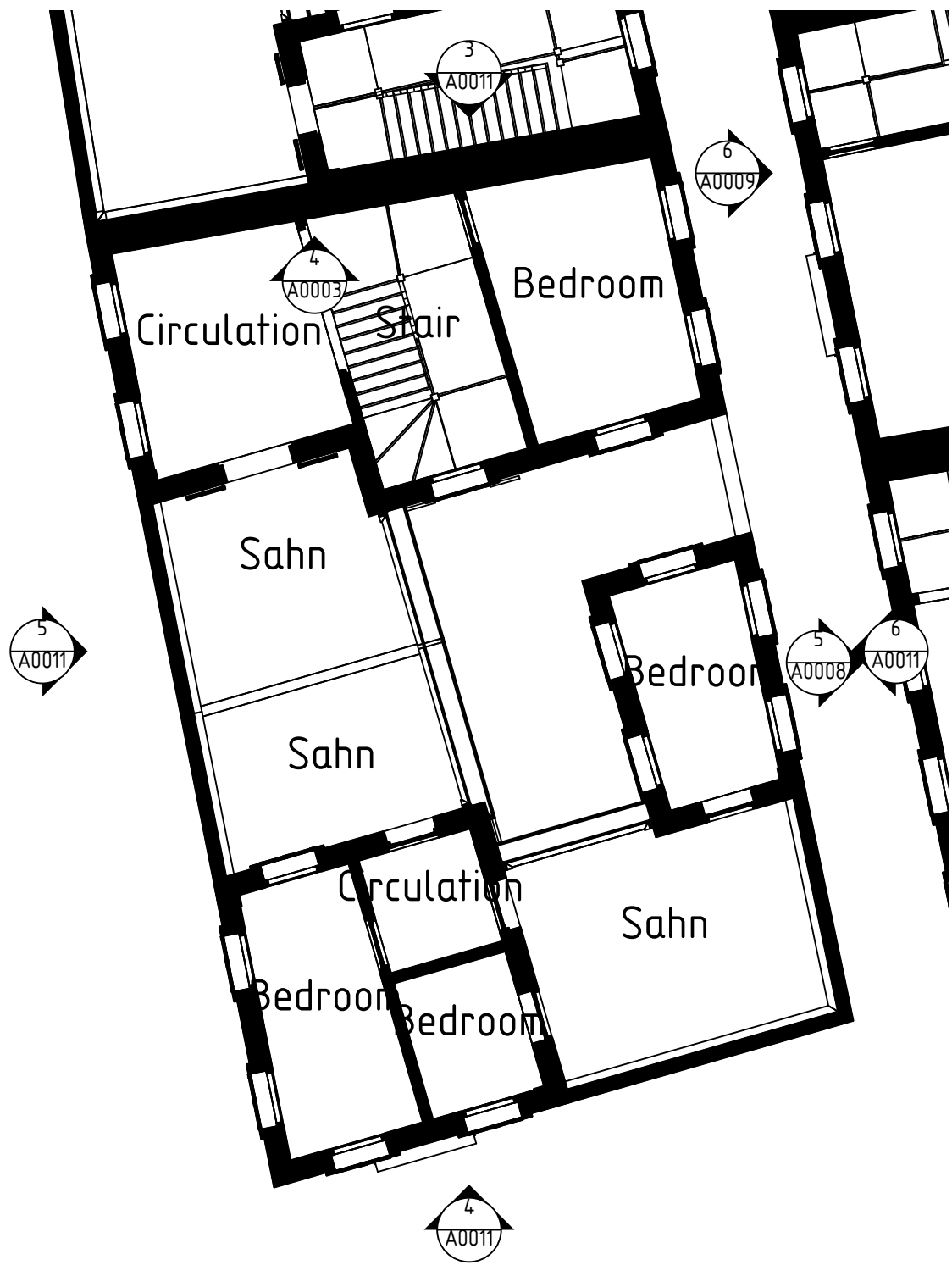
2 plot-9 1 1:100
