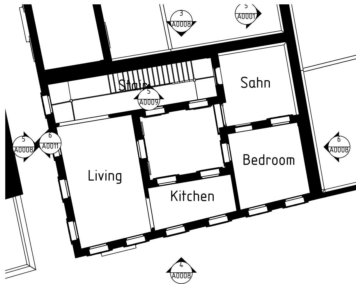
2 plot-6 1 1:100
